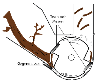
Duplex-Messertrommel
