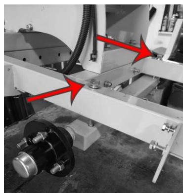
Achse verschrauben
